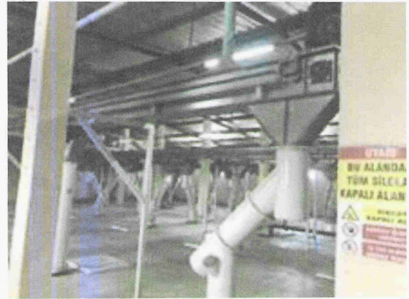
Zincirli Konveyör
